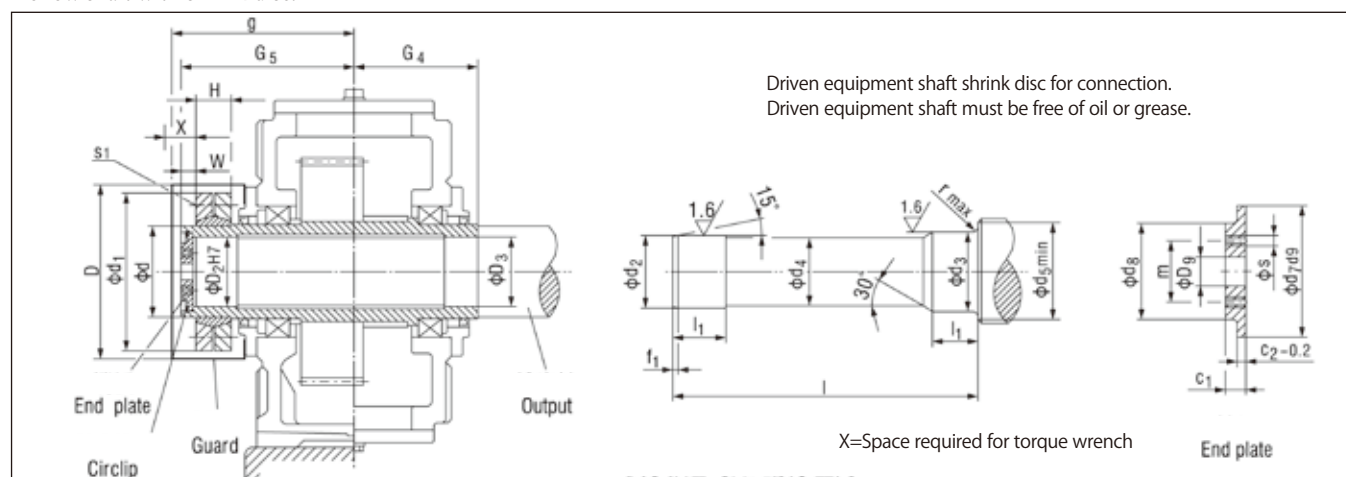
Gear unit size Driven equipment shaft 2) End plate Circlip Hollow shaft Shrink disk 1) Bolt Protection cover d 2 d 3 d 4 d 5 f 1 l l 1 r c 1 c 2 d 7 d 8 D 9 m s Qty. D 2 D 3 G 4 G 5 Type d d 1 H W s 1 D g 4 85 g6 85 h6 84.5 95 4 326 48 2 17 7 90 70 22 50 M 8 2 90 x 3 85 85 140 205 SP2-110 110 185 49 20 M 12 235 220 5 100 g6 100 h6 99.5 114 5 383 53 2 20 8 105 80 26 55 M 10 2 105 x 4 100 100 165 240 SP2-125 125 215 53 20 M 12 275 255 6 110 g6 110 h6 109.5 124 5 383 58 3 20 8 115 85 26 60 M 10 2 115 x 4 110 110 165 240 SP2-140 140 230 58 20 M 14 285 255 7 120 g6 120 h6 119.5 134 5 453 68 3 20 8 125 90 26 65 M 12 2 125 x 4 120 120 195 280 SP2-155 155 263 62 23 M 14 330 295 8 130 g6 130 h6 129.5 145 6 458 73 3 20 8 135 100 26 70 M 12 2 135 x 4 130 130 195 285 SP2-165 165 290 68 23 M 16 340 300 9 140 g6 140 m6 139.5 160 6 539 82 4 23 10 150 110 33 80 M 12 2 150 x 4 140 140 235 330 SP2-175 175 300 68 28 M 16 360 345 10 150 g6 150 m6 149.5 170 6 559 92 4 23 10 160 120 33 90 M 12 2 160 x 4 150 150 235 350 SP2-200 200 340 85 28 M 16 395 365 11 165 f6 165 m6 164.5 185 7 644 112 4 23 10 175 130 33 90 M 12 2 175 x 4 165 165 270 400 SP2-220 220 370 103 30 M 20 435 420 12 180 f6 180 m6 179.5 200 7 649 122 4 23 10 190 140 33 100 M 16 2 190 x 4 180 180 270 405 SP2-240 240 405 107 30 M 20 450 420 13 190 f6 190 m6 189.5 213 7 789 137 5 23 10 200 150 33 110 M 16 2 200 x 4 190 190 335 480 SP2-260 260 430 119 30 M 20 500 505 14 210 f6 210 m6 209.5 233 8 784 147 5 28 14 220 170 33 130 M 16 2 220 x 5 210 210 335 480 SP2-280 280 460 132 30 M 20 525 505 15 230 f6 230 m6 229.5 253 8 899 157 5 28 14 240 180 39 140 M 16 2 240 x 5 230 230 380 550 SP2-300 300 485 140 35 M 24 575 575 16 240 f6 240 m6 239.5 263 8 899 157 5 28 14 250 190 39 150 M 20 2 250 x 5 240 240 380 550 SP2-320 320 520 140 35 M 24 595 575 17 250 f6 250 m6 249.5 278 8 982 177 5 30 14 265 200 39 150 M 20 2 265 x 5 250 250 415 600 SP2-340 340 570 155 35 M 24 615 630 18 280 f6 280 m6 279.5 306 9 982 177 5 30 14 290 210 39 160 M 20 2 290 x 5 280 280 415 600 SP2-360 360 590 162 35 M 24 635 625 19 285 f6 285 m6 284.5 316 9 1100 187 5 32 15 300
